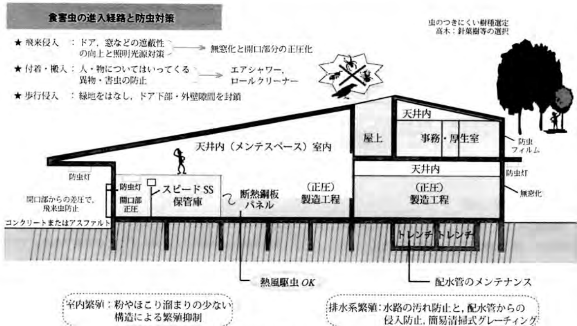
図1 食害虫の工場への侵入経路と防虫対策例
