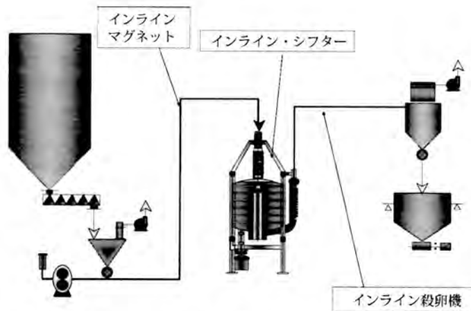
図2 インライン異物除去装置のフロー例
